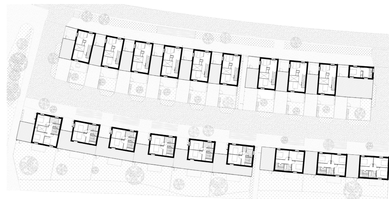
Étage - R+1
